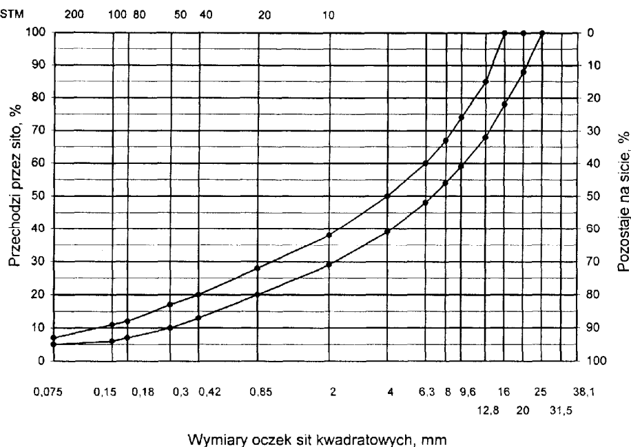
Rys. 4. Krzywe graniczne uziarnienia mieszanki mineralnej BA od 0 do 20 mm do warstwy ścieralnej nawierzchni
